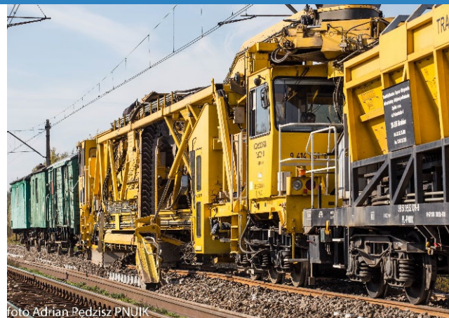
Oczyszczarka tuczni OT 84.00
